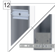
Elementy wzmacniające konstrukcję ościeznicy z kotwami montażowymi lub bez 11. Ościeznica 10/54, 11/54 12. Ościeznica 15/54
