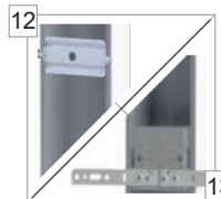
12 Elementy wzmacniające konstrukcję ościeżnicy z kotwami montażowymi lub bez 13. Ościeżnica 10/54,11/54 13. Ościeżnica 15/54
