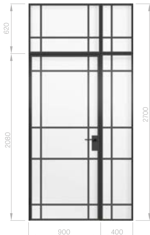
LOFT ART 2
