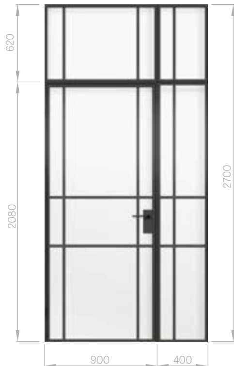
LOFT ART 1
