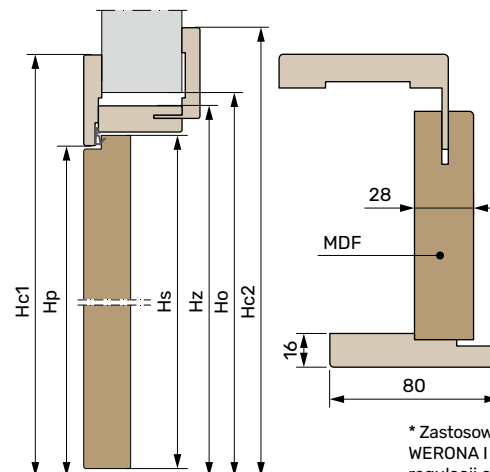
Panel pojedynczy
