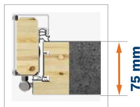
Ościeżnica DUOTHERM 75
