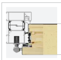
Ościeżnica ALUTHERM 75
