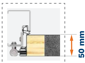
Ościeżnica PERFOTHERM 50*
