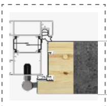
Ościeżnica ALUTHERM 75*
