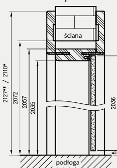
Przekrój pionowy drzwi szklanych z ORC
