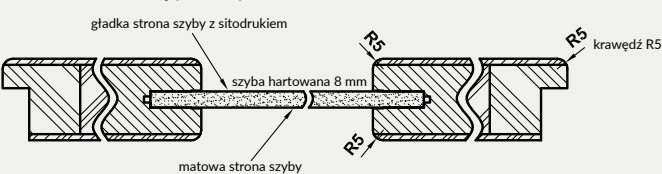
Przekrój poziomy drzwi VETRO B5, B10-B11
