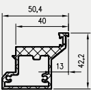
Profil DRE do drzwi z odwróconą przylgą otwieranych do wewnątrz
