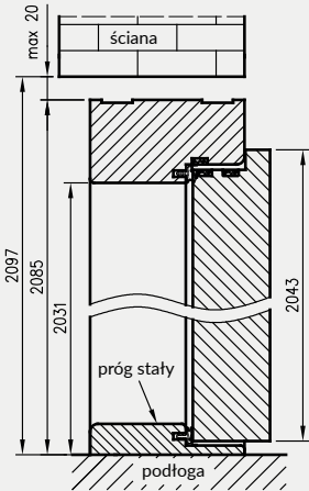
Ościeznica drewniana do drzwi Athos z progiem stałym
