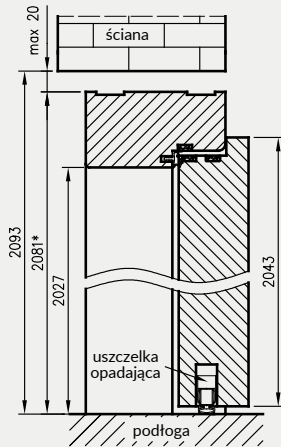
Ościeznica drewniana do drzwi Athos z uszczelką opadającą*
