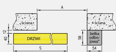
NS - przekrój poziomy (system lewy)
