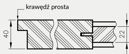
Przekrój poziomy drzwi Elsa
