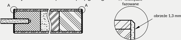
Przekrój ramiaka skrzydła bezprzylgowego
