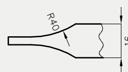
profil płyciny MDF 16 mm (Piano 1, 2, 5, 6)
