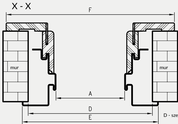
Profil ościeżnicy
