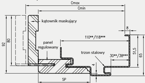
Profil ościeżnicy
