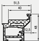
Profil do drzwi z odwróconą przylgą otwieranych do wewnątrz
