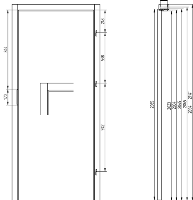
wymiar w przypadku OW
