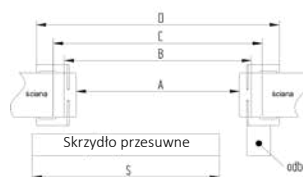
System przesuwny naścienny z zabudową
