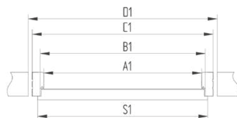
Wymiary ościeznic stałych (OS)
