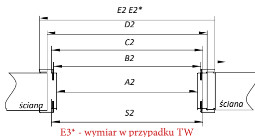
E3* - wymiar w przypadku TW
