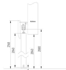
System przesuwny naścienny bez zabudowy
