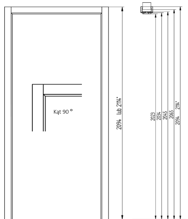
wymiar w przypadku TW
