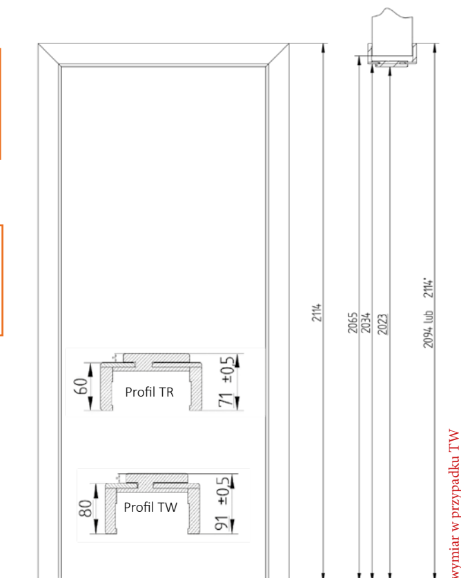
Opaska kątowa TW
