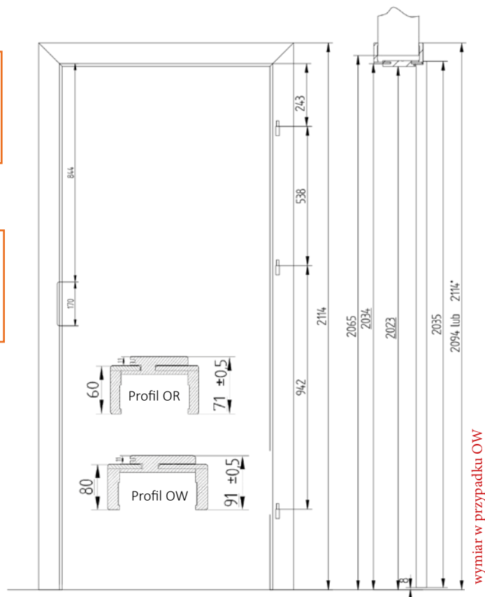
Opaska kątowa OW
