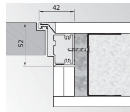
odwrotna przylga (otwierane do wewnątrz)
